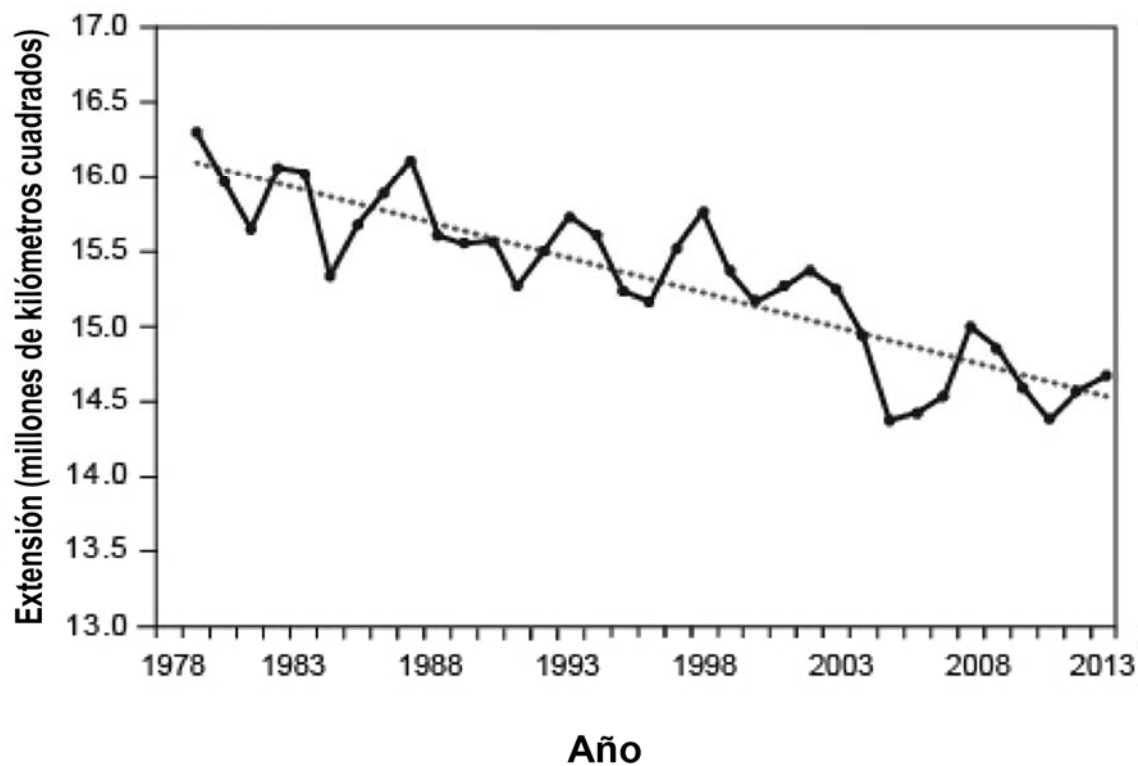
Extensión promedio mensual de hielo en el océano Ártico Febrero 1979 - 2013
